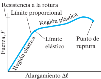
FIGURA 12-15 Fuerza aplicada versus alargamiento para un metal típico sometido a tensión.
