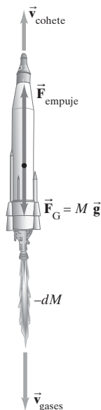
FIGURA 9-35 Ejemplo 9-20; \vec{v}_{\text{rel}} = \vec{v}_{\text{gases}} - \vec{v}_{\text{cohete}} . M es la masa del cohete en cualquier instante y disminuye hasta que se quema el combustible.
