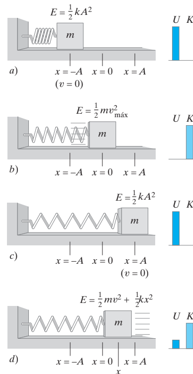
FIGURA 14-10 La energía cambia de energía cinética a energía potencial y viceversa, cuando el resorte oscila. Las gráficas de barras para la energía (a la derecha) se describen en la sección 8-4.
