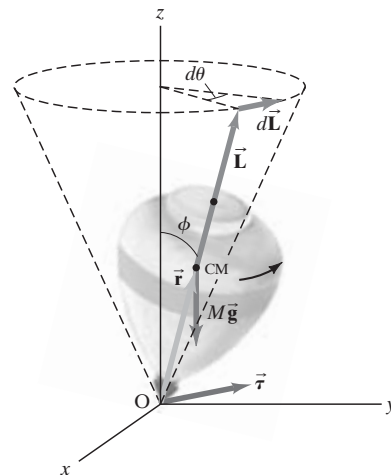
FIGURA 11-23 Trompo en rotación.
