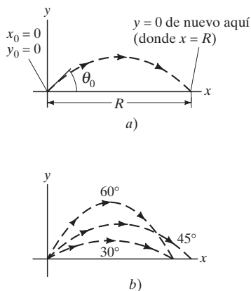
FIGURA 3-27 Ejemplo 3-10. a) El alcance R de un proyectil; b) generalmente hay dos ángulos \theta_0 que darán el mismo alcance. ¿Puede usted demostrar que si un ángulo es \theta_{01} , el otro será \theta_{02} = 90^\circ - \theta_{01} ?
