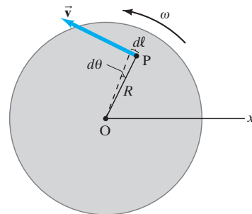
FIGURA 10-5 Un punto P sobre una rueda en rotación tiene una velocidad lineal \vec{v} en cualquier momento.
