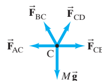
e) Pasador C
