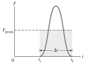
FIGURA 9-10 La fuerza promedio F_{\text{prom}} que actúa sobre un intervalo de tiempo muy breve \Delta t da el mismo impulso ( F_{\text{prom}} \Delta t ) que la fuerza real.
