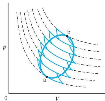
FIGURA 20-12 Cualquier ciclo reversible se puede aproximar como una serie de ciclos de Carnot. (Las líneas punteadas representan isothermas).
