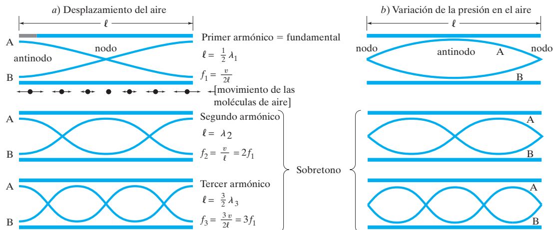
FIGURA 16-11 Gráfica de los tres modos más simples de vibración (ondas estacionarias) para un tubo uniforme abierto en ambos extremos (“tubo abierto”). Estos modos más simples de vibración se muestran en a), a la izquierda, en términos del movimiento del aire (desplazamiento); y en b), a la derecha, en términos de presión del aire. Cada gráfica, muestra el formato de onda en dos momentos: A y B, separados medio periodo. El movimiento real de las moléculas en el caso fundamental, se muestra justo abajo del tubo arriba a la izquierda.
