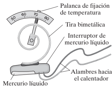
FIGURA 17-18 Un termostato (pregunta 10).
