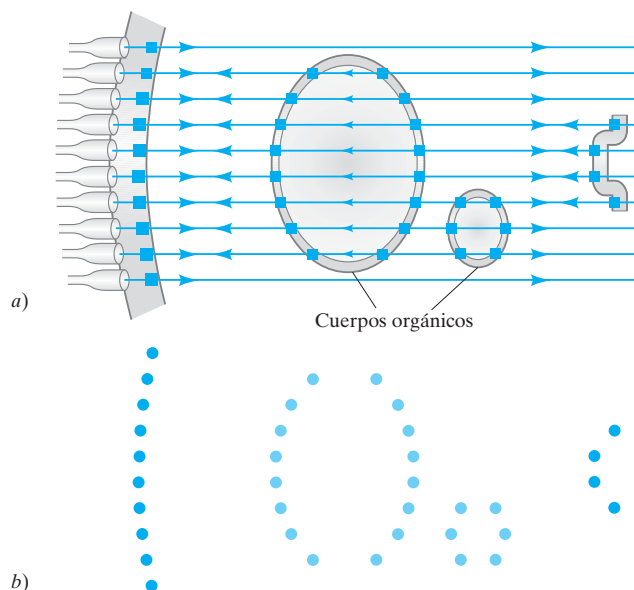
FIGURA 16-26 a) Se forman diez trazas a través del abdomen moviendo el transductor, o usando varios transductores. b) Los ecos se grafican como puntos para producir la imagen. Trazas espaciadas más cercanamente darían una imagen más detallada.
