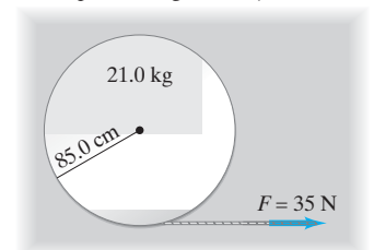
FIGURA 10-71 Problema 100, viendo el disco hacia abajo.
