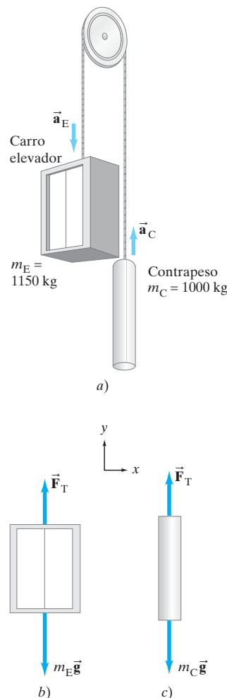
FIGURA 4-23 Ejemplo 4.13. a ) Máquina de Atwood en forma de un sistema elevador-contrapeso. b ) y c ) Diagramas de cuerpo libre para los dos objetos.
