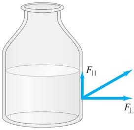
FIGURA 13-2 Si hubiera una componente de la fuerza paralela a la superficie sólida del recipiente, el líquido se movería en respuesta a ella. Para un líquido en reposo, F_{\parallel} = 0 .
