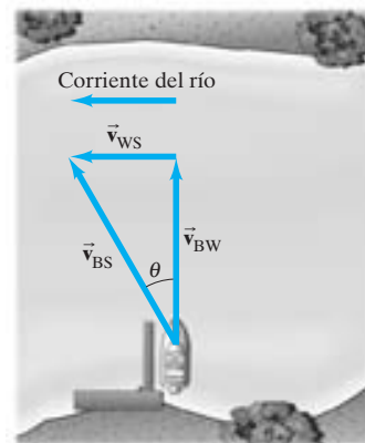
FIGURA 3-34 Ejemplo 3-15. Un bote que cruza directamente un río cuya corriente se mueve a 1.20 \text{ m/s} .
