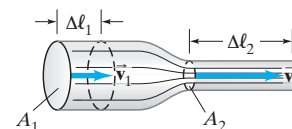
FIGURA 13-22 Flujo de un fluido a través de un tubo de diámetro variable.
