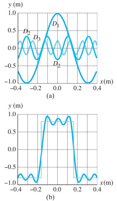
FIGURA 15-17 Ejemplo 15-7. Generación de una onda cuadrada.
