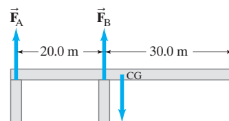
FIGURA 12-7 Un voladizo. Los vectores de fuerza que se muestran son hipotéticos: las direcciones reales pueden ser opuestas a las direcciones mostradas.
