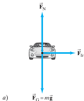
FIGURA 5-23 Ejemplo 5-14. Fuerzas sobre un auto en una curva sobre un camino plano. a) Vista frontal. b) Vista superior.
