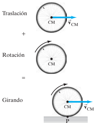
FIGURA 10-32 Una rueda que gira sin deslizamiento puede considerarse como una traslación pura de la rueda como un todo con velocidad \vec{v}_{\text{CM}} más una rotación pura alrededor del CM.
