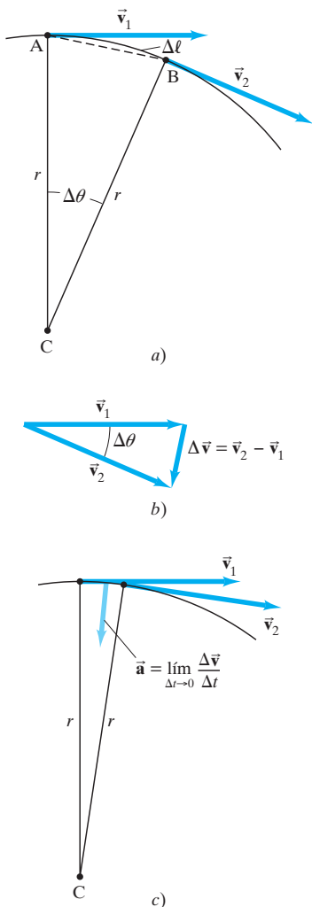
FIGURA 5-11 Determinación del cambio en velocidad, \Delta \vec{v} , para una partícula que se mueve en una trayectoria circular. La longitud \Delta \ell es la distancia a lo largo del arco, desde A hasta B.
