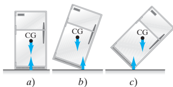
FIGURA 12-12 Equilibrio de un refrigerador que descansa sobre una superficie plana.
