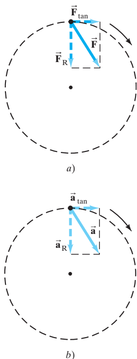
FIGURA 5-25 La rapidez de un objeto que se mueve en círculo cambia si la fuerza que se ejerce sobre él tiene una componente tangencial, F_{\text{tan}} . La parte a) muestra la fuerza \vec{F} y sus componentes vectoriales; la parte b) muestra el vector aceleración y sus componentes vectoriales.
