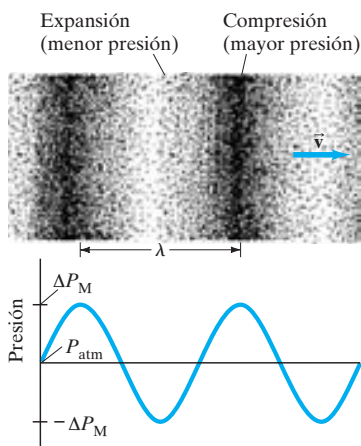
FIGURA 16-2 Onda sonora longitudinal que viaja hacia la derecha, y su representación gráfica en términos de presión.
