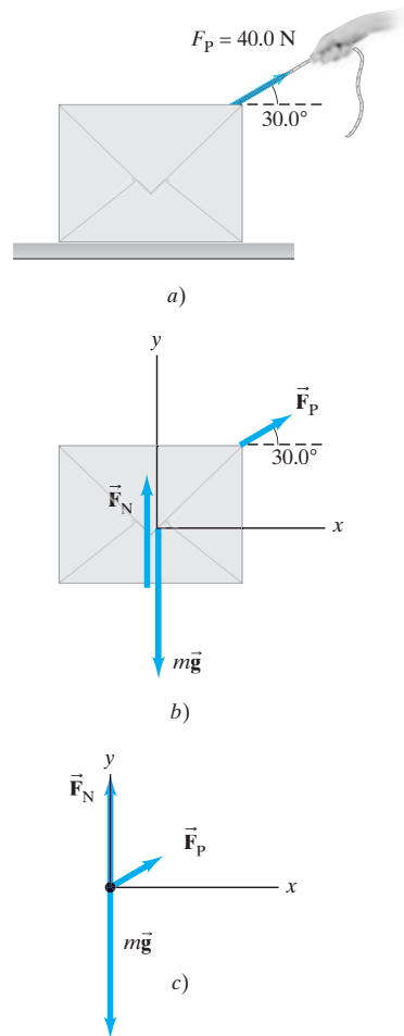
FIGURA 4-21 a) Jalando la caja, ejemplo 4-11; b) es el diagrama de cuerpo libre para la caja; y c) es el diagrama de cuerpo libre considerando que todas las fuerzas actúan sobre un punto (sólo movimiento traslacional, que es lo que tenemos aquí).
