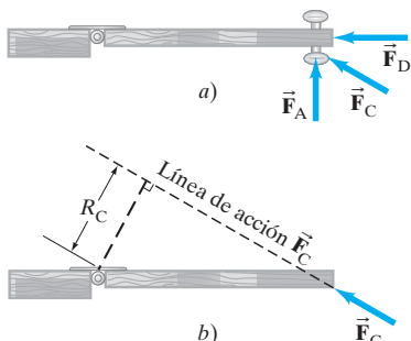
FIGURA 10-13 a) Fuerzas que actúan a diferentes ángulos en la manija de la puerta. b) El brazo de palanca se define como la distancia perpendicular desde el eje de rotación (la bisagra) hasta la línea de acción de la fuerza.
