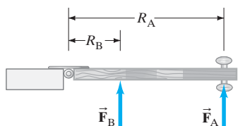
FIGURA 10-11 Vista superior de una puerta. Aplicación de la misma fuerza con brazos de palanca diferentes, R_A y R_B . Si R_A = 3R_B , entonces para crear el mismo efecto (aceleración angular), F_B necesita ser tres veces F_A , o F_A = \frac{1}{3}F_B .
