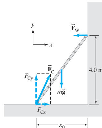
FIGURA 12-10 Una escalera apoyada contra una pared. Ejemplo 12-6.
