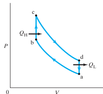
FIGURA 20-8 El ciclo de Otto.
