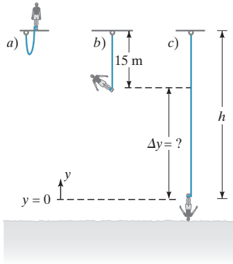
FIGURA 8-47 Problema 103. a) Un individuo a punto de saltar atado a una cuerda bungee . b) Longitud de la cuerda bungee sin estirar. c) Estiramiento máximo de la cuerda.
