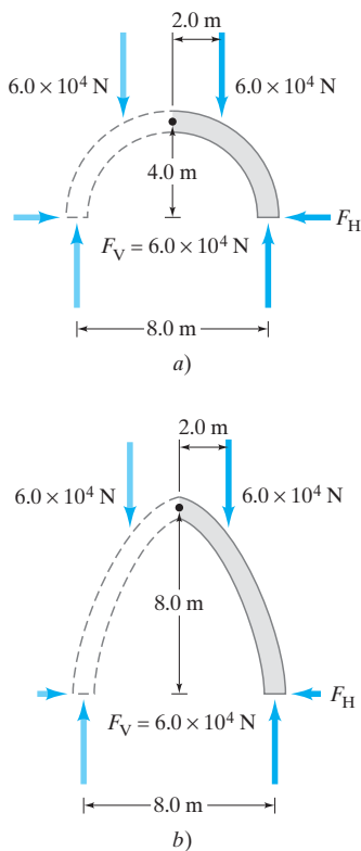
FIGURA 12-36 a) Fuerzas en un arco redondo, comparadas b) con las de un arco apuntado.
