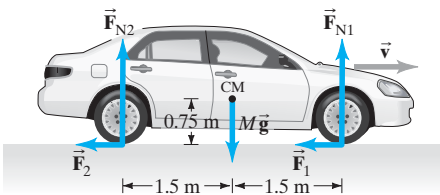
FIGURA 10-39 Fuerzas sobre un automóvil que frena (ejemplo 10-21).
