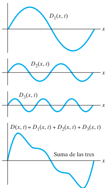
FIGURA 15-16 El principio de superposición para ondas unidimensionales. Una onda compuesta formada a partir de tres ondas sinusoidales de diferentes amplitudes y frecuencias ( f_0 , 2f_0 , 3f_0 ) en cierto instante en el tiempo. La amplitud de la onda compuesta en cada punto del espacio, en cualquier momento, es la suma algebraica de las amplitudes de las ondas componentes. Las amplitudes se muestran exageradas; para que se sostenga el principio de superposición, las amplitudes deben ser pequeñas comparadas con las longitudes de onda.
