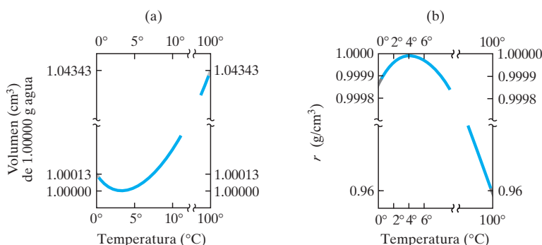
FIGURA 17-12 Comportamiento del agua como función de la temperatura cerca de 4°C. a) Volumen de 1.00000 g de agua, como función de la temperatura. b) Densidad versus temperatura. [Note el cambio de escala en cada eje].
