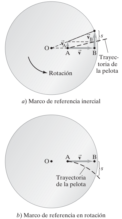
FIGURA 11-26 Origen del efecto Coriolis. Observando hacia abajo una plataforma que gira, a) vista desde un marco de referencia inercial, que no gira; y b) vista desde una plataforma en rotación como marco de referencia.
