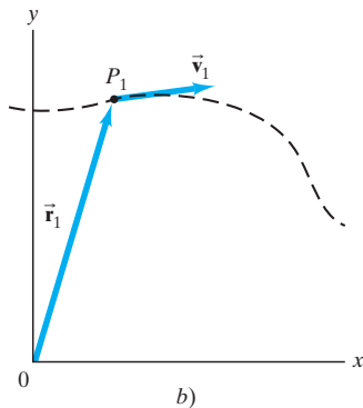
FIGURA 3-17 a) Cuando tomamos \Delta t y \Delta \vec{r} cada vez más pequeño [compare con la figura 3-16], vemos que la dirección de \Delta \vec{r} y de la velocidad instantánea ( \Delta \vec{r}/\Delta t , cuando \Delta t \rightarrow 0 ) es b) tangente a la curva en P_1 .
