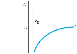
FIGURA 8-20 Energía potencial gravitacional graficada en función de r , la distancia desde el centro de la Tierra. Válida sólo para puntos r > r_E el radio terrestre.
