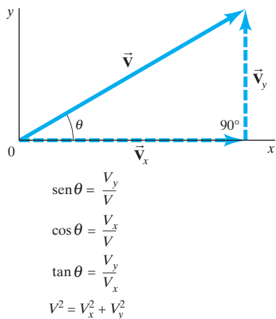
FIGURA 3-11 Determinación de las componentes de un vector usando funciones trigonométricas.
