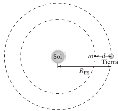
FIGURA 6-19 Cálculo de la posición del punto de Lagrange L1 para un satélite que puede permanecer a lo largo de la línea recta entre el Sol y la Tierra, a una distancia d de la Tierra. Es decir, una masa m en L1 tiene el mismo periodo alrededor del Sol que la Tierra. (No está a escala).
