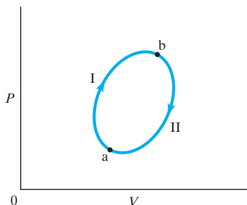
FIGURA 20-13 La integral, \oint dS , de la entropía para un ciclo reversible es cero. Por lo tanto, la diferencia en la entropía entre los estados a y b, S_b - S_a = \int_a^b dS , es la misma para la trayectoria I que para la trayectoria II.
