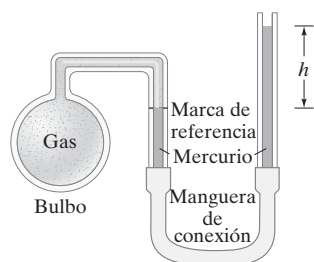
FIGURA 17-8 Termómetro de gas a volumen constante.
