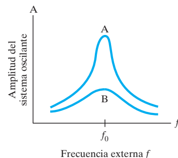
FIGURA 14-23 Resonancia para sistemas ligeramente amortiguados (A) y fuertemente amortiguados (B). (Véase en la figura 14-26 una gráfica más detallada).
