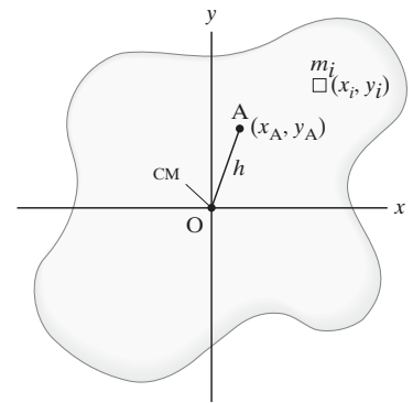
FIGURA 10-26 Derivación del teorema de los ejes paralelos.
