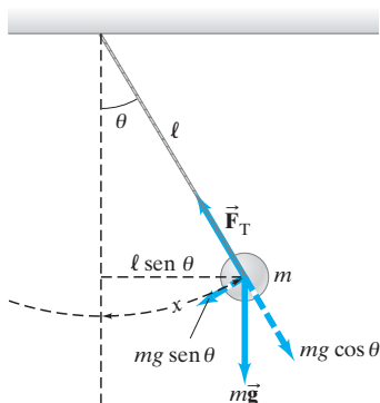
FIGURA 14-14 Péndulo simple.
