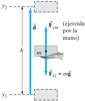
FIGURA 8-4 Una persona ejerce una fuerza hacia arriba F_{\text{ext}} = mg para levantar un ladrillo de y_1 a y_2 .
