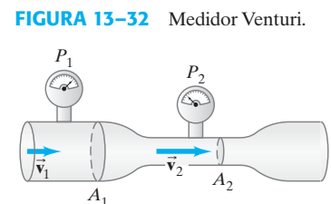
FIGURA 13-32 Medidor Venturi.
