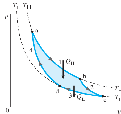
FIGURA 20-7 El ciclo de Carnot. Las máquinas térmicas trabajan en un ciclo, y el ciclo para la máquina de Carnot comienza en el punto a sobre este diagrama PV . (1) Primero, el gas se expande isotérmicamente, con la adición de calor Q_H , a lo largo de la trayectoria ab a temperatura T_H . (2) A continuación el gas se expande adiabáticamente de b a c , no se intercambia calor, sino que la temperatura disminuye a T_L . (3) Luego, el gas se comprime a temperatura constante T_L , trayectoria cd , y fluye hacia fuera calor Q_L . (4) Finalmente, el gas se comprime adiabáticamente, trayectoria da , de regreso a su estado original. En realidad, no existe ninguna máquina de Carnot, pero como planteamiento teórico desempeñó un importante papel en el desarrollo de la termodinámica.
