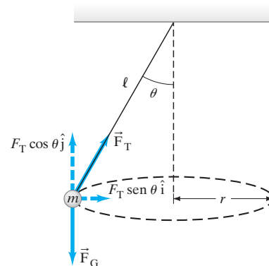
FIGURA 5-20 Ejemplo 5-13. Péndulo cónico.
