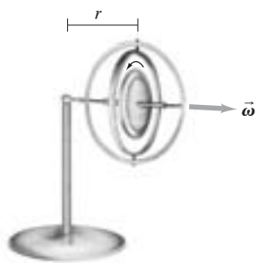
FIGURA 11-24 Un giroscopio de juguete.
