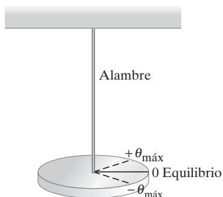
FIGURA 14-18 Péndulo de torsión. El disco oscila en MAS entre \theta_{\text{máx}} y -\theta_{\text{máx}} .
