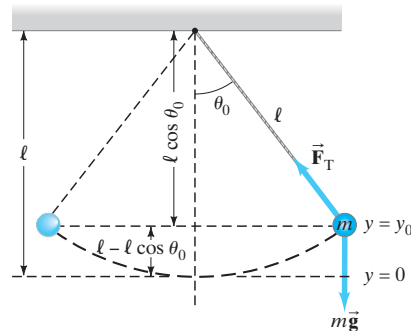
FIGURA 8-14 Ejemplo 8-9: un péndulo simple; y se mide como positiva hacia arriba.
