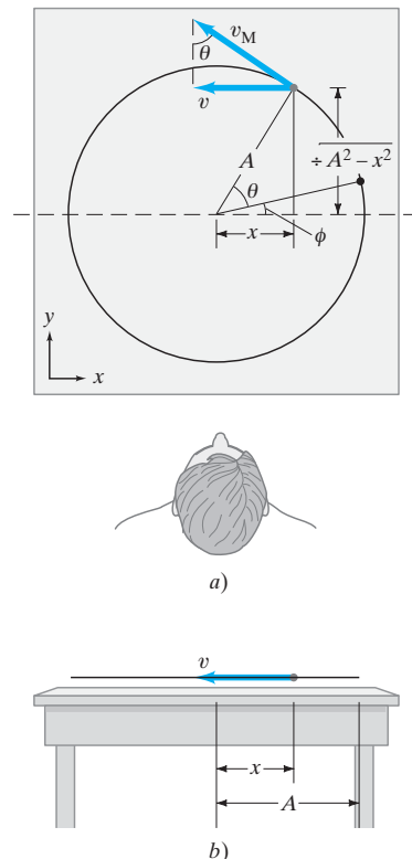
FIGURA 14-12 Análisis de un movimiento armónico simple como una vista lateral b) de un movimiento circular a).
