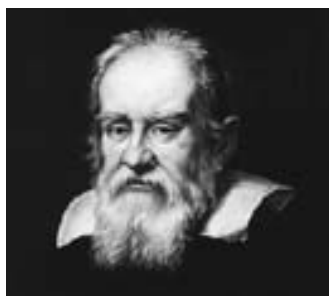
FIGURA 2-25 Galileo Galilei (1564-1642).
