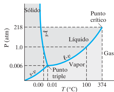
FIGURA 18-5 Diagrama de fase para el agua (las escalas no son lineales).
