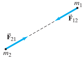
FIGURA 6-7 Por la tercera ley de Newton, la fuerza gravitacional sobre la partícula 1 ejercida por la partícula 2, \vec{\mathbf{F}}_{12} , tiene la misma magnitud y dirección, pero sentido opuesto a la fuerza gravitacional que ejerce la partícula 1 sobre la partícula 2, \vec{\mathbf{F}}_{21} ; es decir, \vec{\mathbf{F}}_{21} = -\vec{\mathbf{F}}_{12} .
