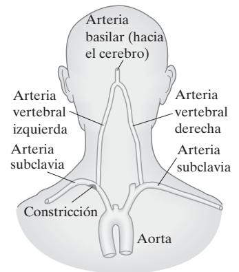
FIGURA 13-31 Parte posterior de la cabeza que muestra las arterias que van al cerebro y a los brazos. La alta velocidad de la sangre que pasa por la constricción en la arteria subclavia izquierda causa baja presión en la arteria vertebral izquierda, en la que puede generarse un flujo inverso (hacia abajo), que provoca un AIT, es decir, un menor suministro de sangre al cerebro.
