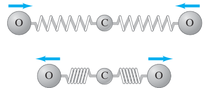
FIGURA 14-43 Problema 86, la molécula de CO 2 .
