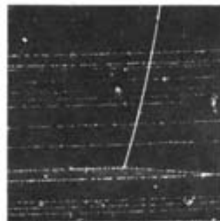
FIGURA 9-20 Fotografía de una colisión protón-protón en una cámara de burbujas de hidrógeno (dispositivo que hace visibles las trayectorias de partículas elementales). Las líneas múltiples representan los protones que entran y pueden golpear a los protones del hidrógeno en la cámara.
