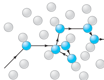
FIGURA 18-12 Trayectoria en zigzag de una molécula que choca con otras moléculas.
