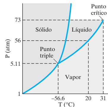
FIGURA 18-6 Diagrama de fase para el dióxido de carbono.
