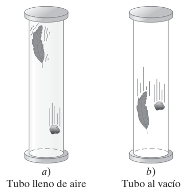
FIGURA 2-28 Una piedra y una pluma se dejan caer simultáneamente a) en el aire y b) en un vacío.
