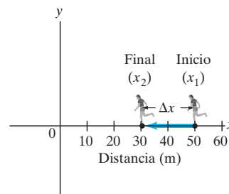
FIGURA 2-7 Ejemplo 2-1. Una persona corre de x_1 = 50.0 \text{ m} a x_2 = 30.5 \text{ m} . El desplazamiento es -19.5 \text{ m} .
