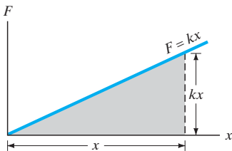
FIGURA 7-11 El trabajo hecho al estirar un resorte una distancia x es igual al área triangular bajo la curva F = kx . El área de un triángulo es \frac{1}{2} \times \text{base} \times \text{altura} , por lo que W = \frac{1}{2}(x)(kx) = \frac{1}{2} kx^2 .
