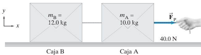
FIGURA 4-22 Ejemplo 4-12. a) Dos cajas, A y B, están conectadas por una cuerda. Una persona jala horizontalmente sobre la caja A con una fuerza F_P = 40.0 N. b) Diagrama de cuerpo libre de la caja A. c) Diagrama de cuerpo libre de la caja B.
