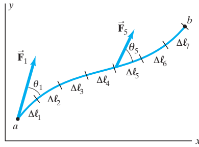
FIGURA 7-8 Una partícula, sobre la que actúa una fuerza variable \vec{F} , se mueve a lo largo de la trayectoria que se muestra del punto a al punto b .
